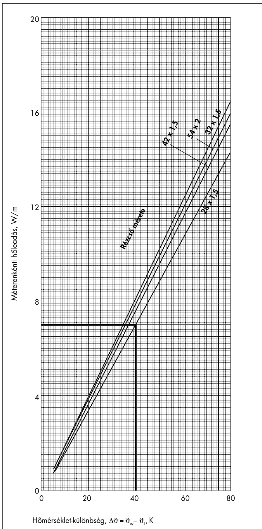
1.1. ábra. Szabadon szerelt bevonatos rézcső méterenkénti hőleadása
