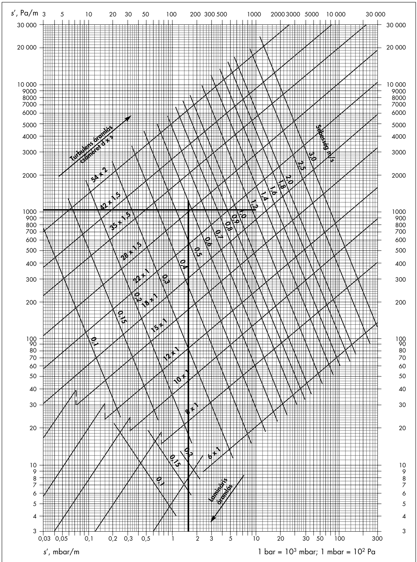
3.2. ábra. Fűtéméretezési nomogram t_{köz} = 60 \text{ }^\circ\text{C}
