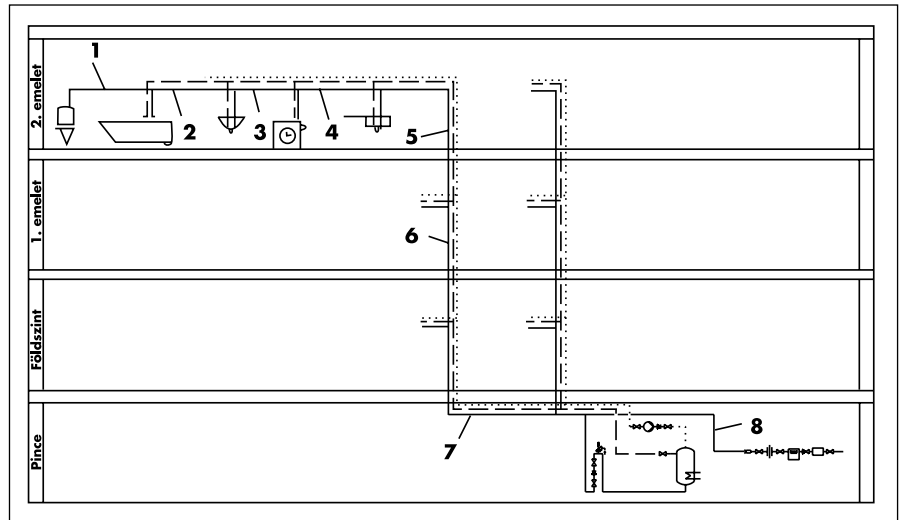
2.1. ábra. Lakóépület vízellátásának függőleges csőterve
