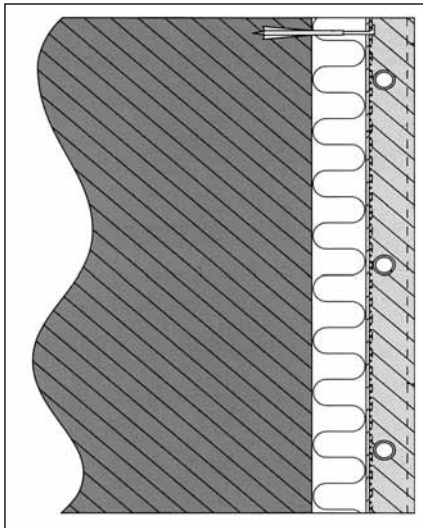
3.8. ábra. Falfűtés elvi kialakítása
