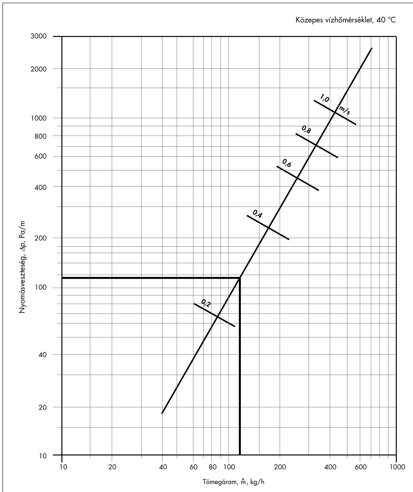
3.6. ábra. Padlófűtési cső fajlagos súrlódási ellenállása (14 x 0,8 mm-es rézcső)
