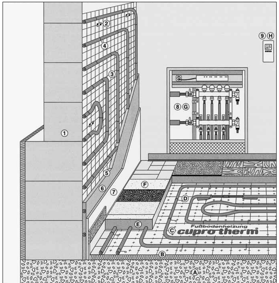
3.11. ábra. Padlófűtés és falfűtés kombinációja
